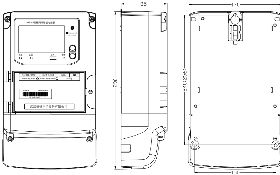
外形示意图
